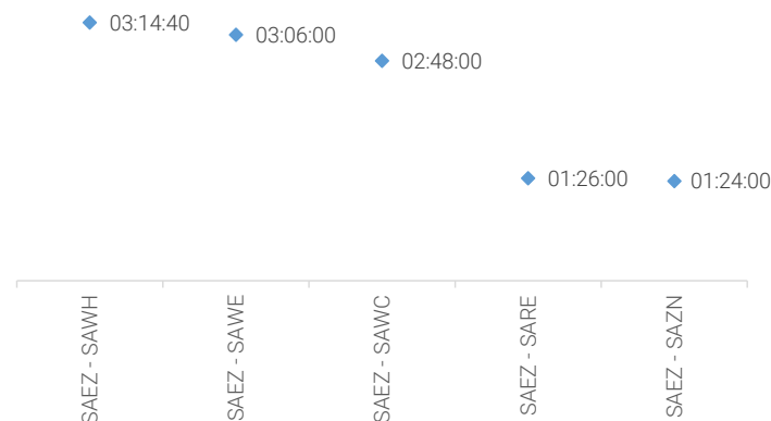
Top 5- Vuelos más Largos del Ranking
