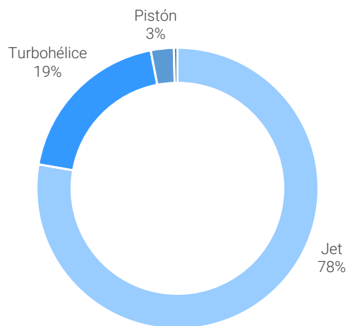
% Aeronaves por Tipo de Motor
