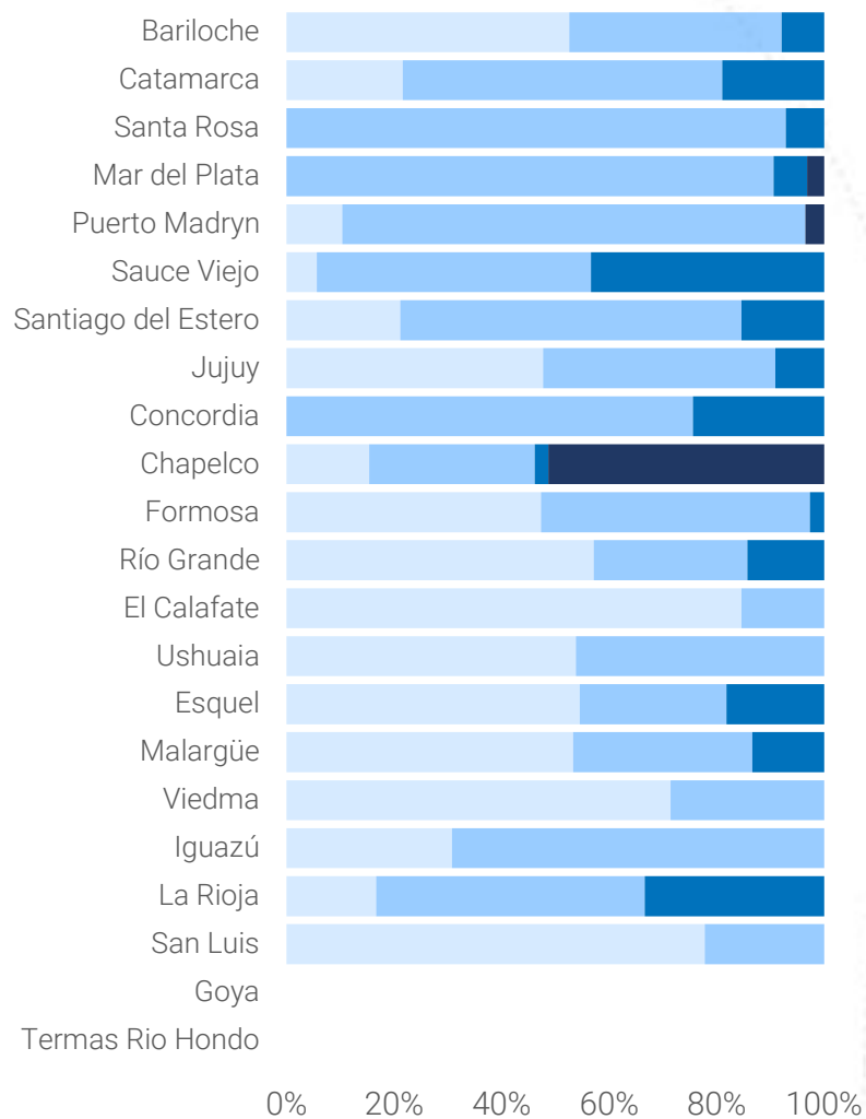
Tipo de Motor por Aeropuerto
