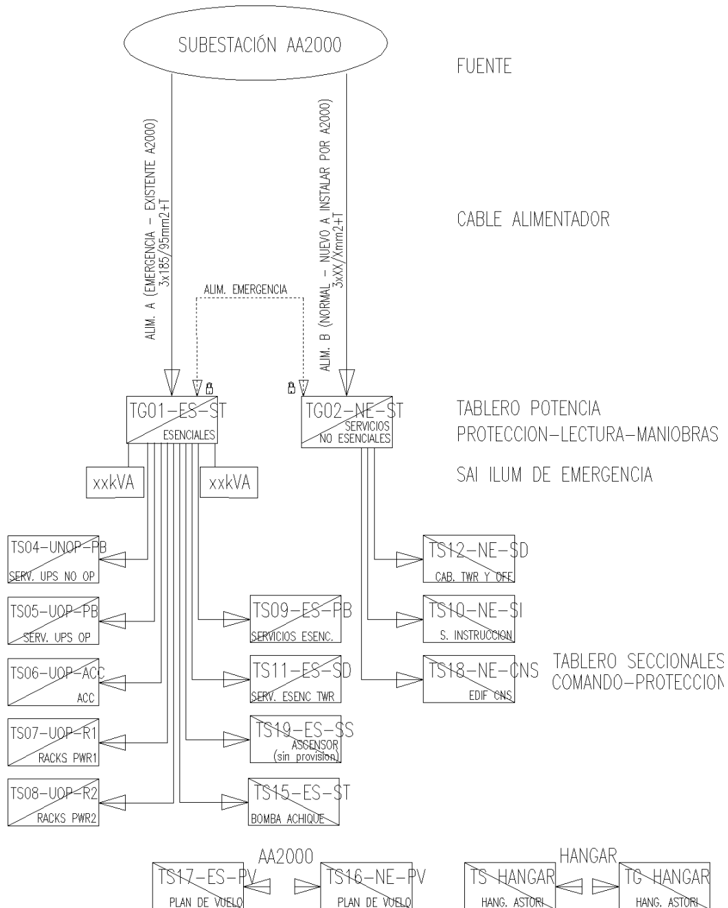
DIAGRAMA ALIMENTACION TWR Y ED. OPERATIVO.
