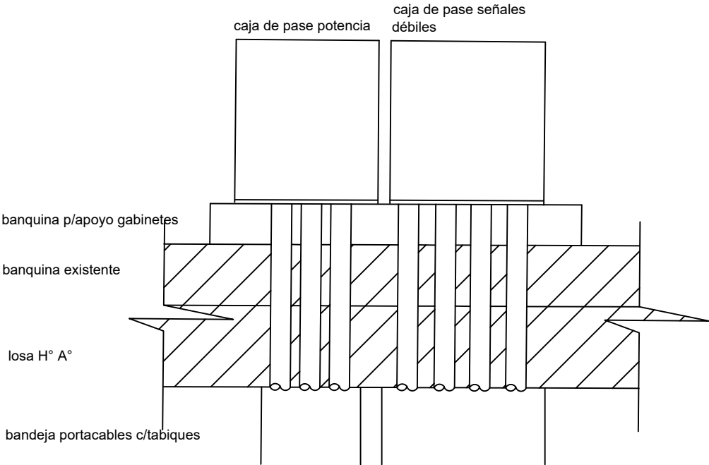
DETALLE CAJAS DE DERIVACION POTENCIA Y SEÑALES DEBILES
